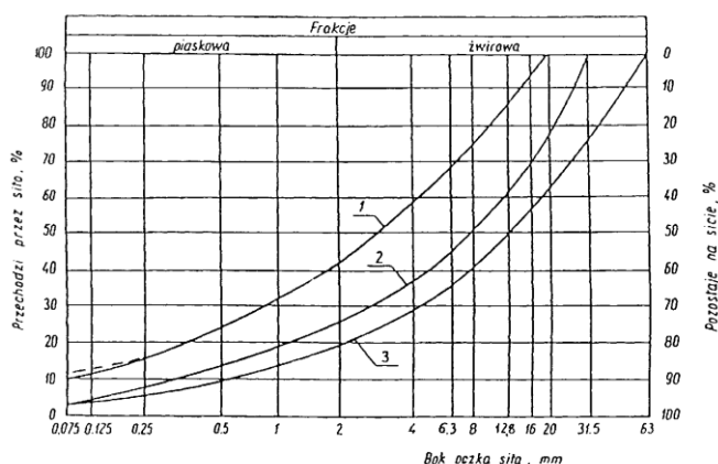
Rysunek kruszyw
