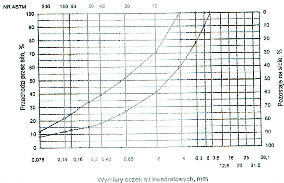
Rys. 3. Krzywe graniczne uziarnienia mieszanki mineralnej BA od 0 do 8 mm, od 0 do 6,3 mm do warstwy ścieralnej nawierzchni drogi o obciążeniu ruchem powierzchni drogi o obciążeniu ruchem KR1 lub KR2
