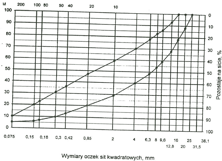
Rys. 1. Krzywe graniczne uziarnienia mieszanki mineralnej BA od 0 do 20 mm do warstwy ścieralnej nawierzchni drogi o obciążeniu ruchem dla KR1 lub KR2
