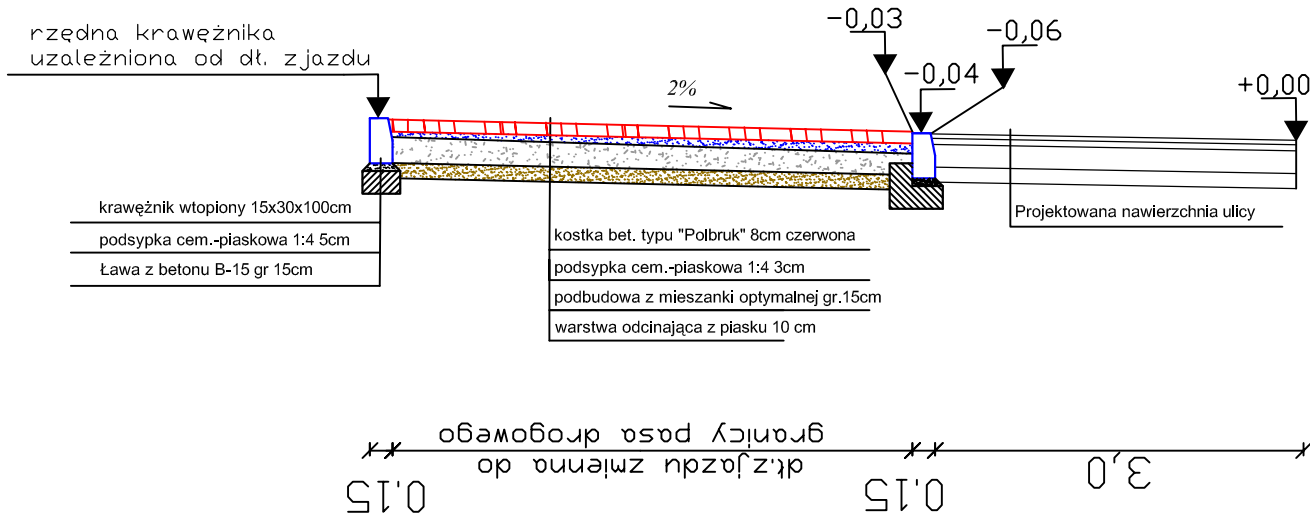
Przekrój A - A (dotyczy przekroju poprzecznego zjazdu)
