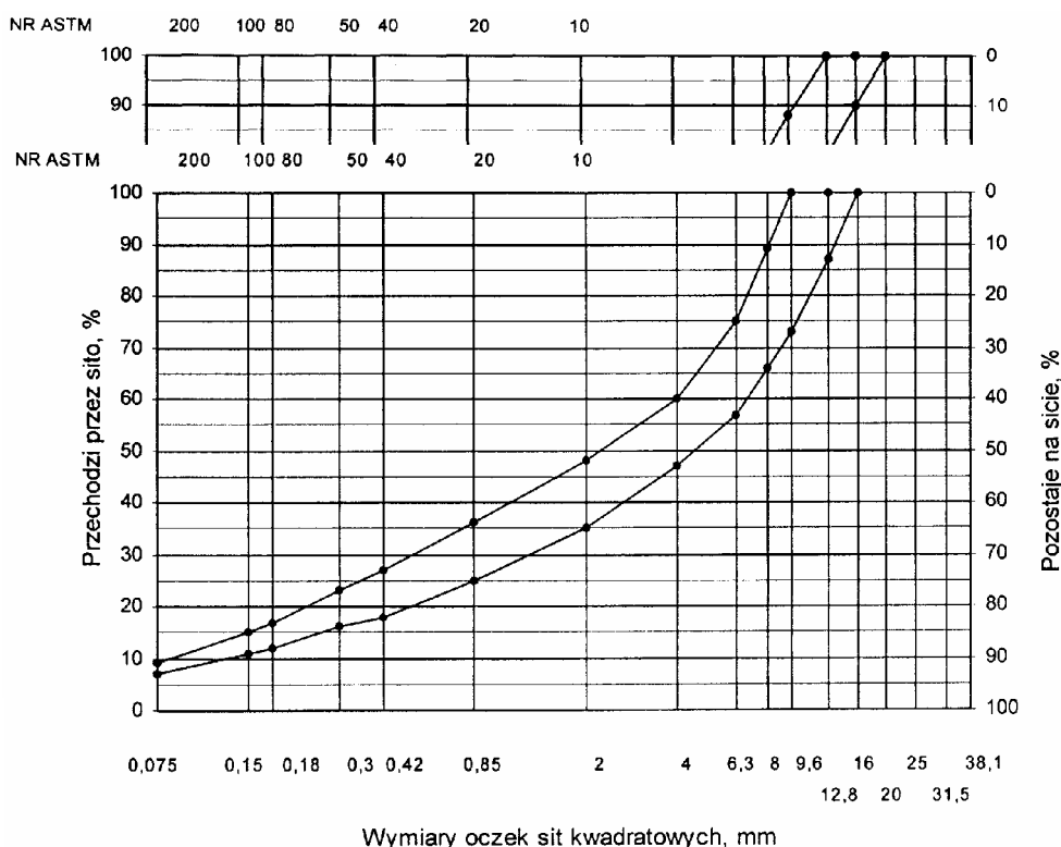
Rys. 6. Krzywe graniczne uziarnienia mieszanki mineralnej BA od 0 do 16 mm do warstwy ścieralnej nawierzchni drogi o obciążeniu ruchem od KR3 do KR6
