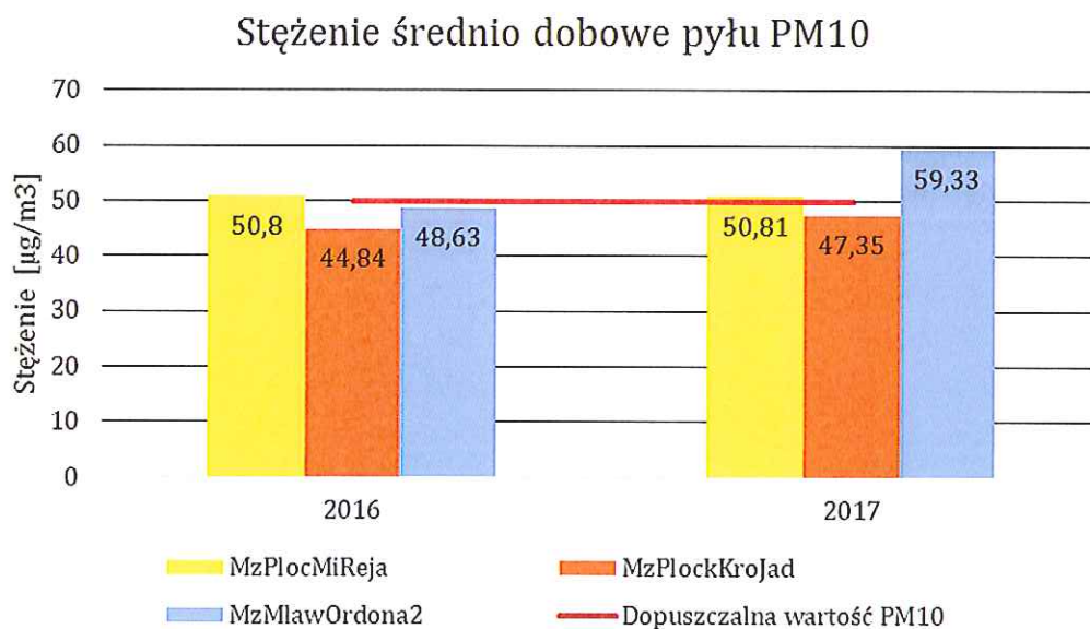
Rysunek 3. Stężenie średnio dobowe pyłu zawieszonego PM10 [źródło: Roczna ocena jakości powietrza w województwie
