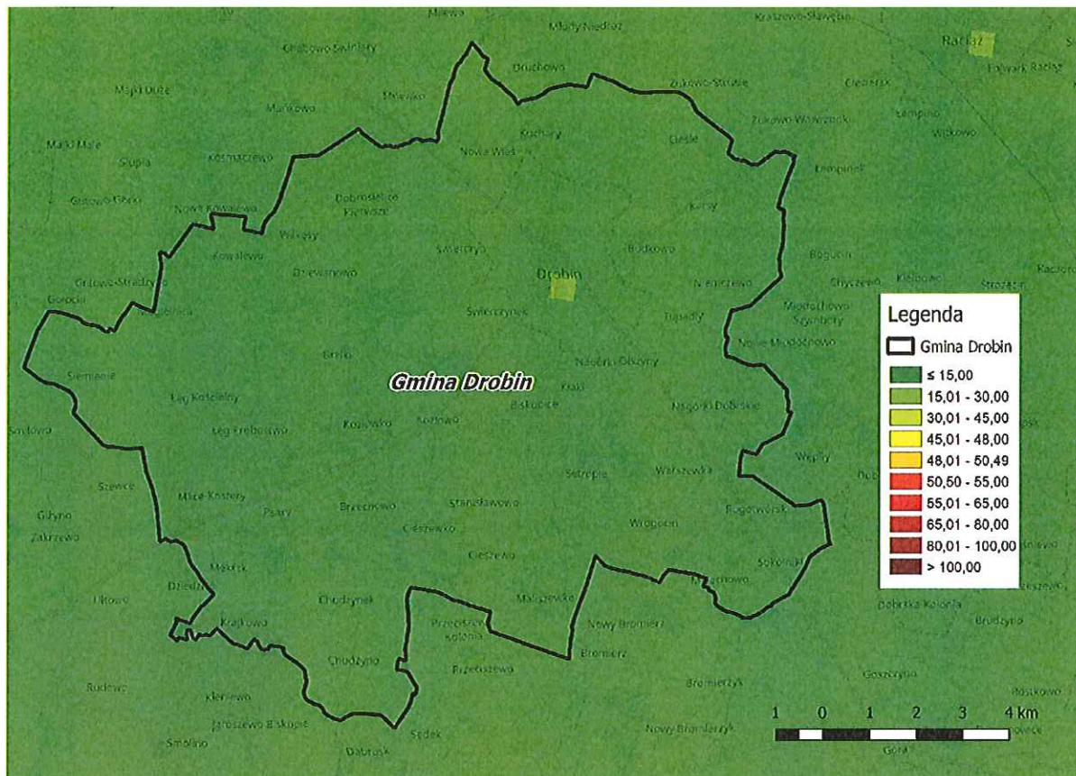
Rysunek 6. Obszary przekroczeń stężeń średniorocznych pyłu zawieszonego PM10 na terenie Gminy Drobin. [opracowanie własne na podstawie http://powietrze.gios.gov.pl/pjp/maps/modeling ]
